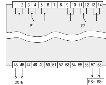
Рис. Б.5. Подключение выходных реле
