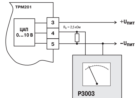
Рис.Е.5. Подключение ВУ типа У
