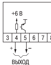
Рис. В.7. Модификация TRM201-X.T
