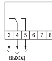
Рис. В.2. Модификация TRM201-X.P
