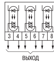
Рис. В.6. Модификация TRM201-X.C3
