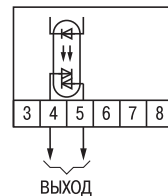
Рис. В.5. Модификация TRM201-X.C
