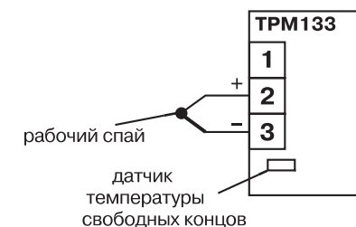
Рис. 3.4. Схема подключения ТП
