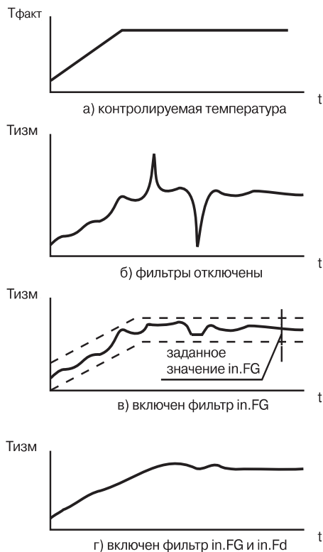
Рис. 3.7. Временные диаграммы работы цифровых фильтров показаний датчика
