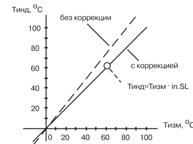
Рис. 3.9. Коррекция "наклон характеристики"
