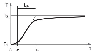
Рис. Д. 3. График переходной функции
