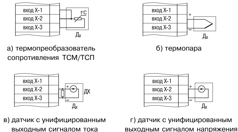
Рис. 3.3. Схемы подключения датчиков
