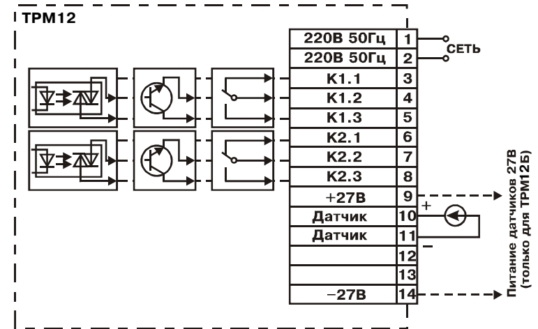
Рис. Г.3. Подключение датчиков с аналоговым выходным сигналом 0...20, 0...5 мА, 4...20 мА, 0...1В
