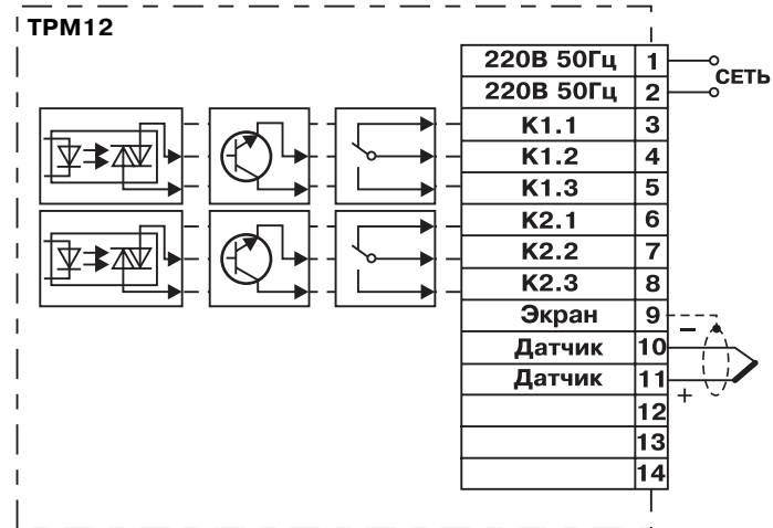
Рис. Г.2. Подключение термоэлектрических преобразователей (термопар)
