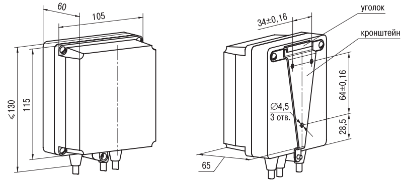
Рис. А.1. Прибор настенного крепления
