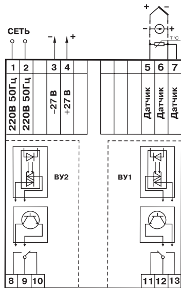
Рис. Г.4. Подключение прибора в DIN-реечном корпусе
