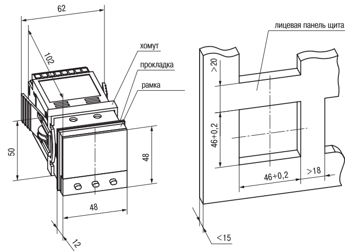
Рис. А. 1. Крепление с помощью крепежного хомута
