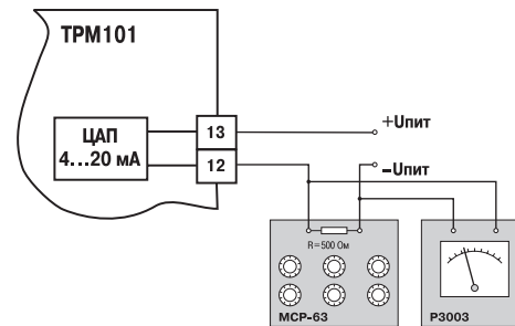
Рис.Е.4 Подключение ВУ1 типа И
