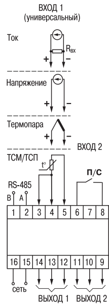
Рис. Б.1. Общая схема подключения
