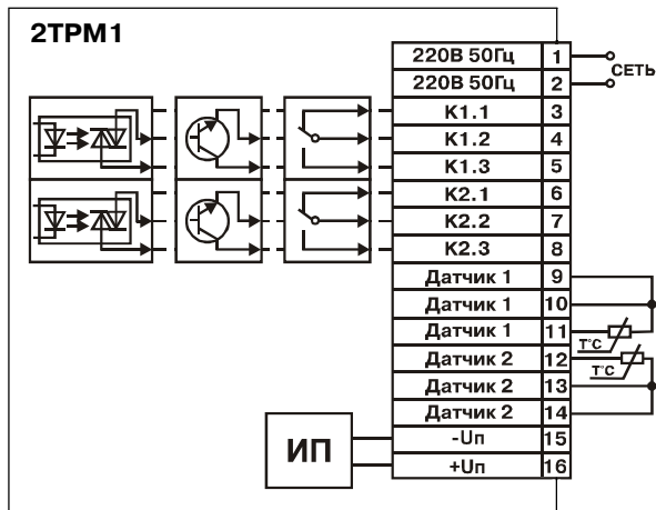
Рис. П2.1. Схема подключения термопреобразователей сопротивления
