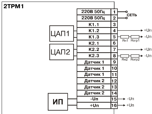
Рис. П2.5. Схема подключения датчиков с аналоговыми выходами
